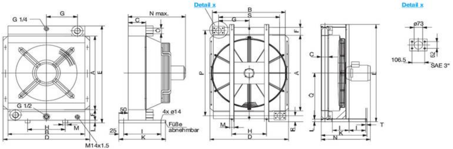
Abmessungen / Bezeichnungen
